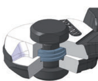
Innenliegende Öffnungsfeder
