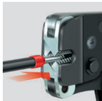
Frontales Einführen von Aderendhülsen z. B. in Schaltschranken
