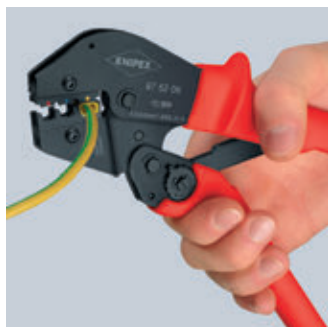
Zweiter Schritt: Jetzt die ganze Hand für den weiteren Crimpvorgang benutzen
