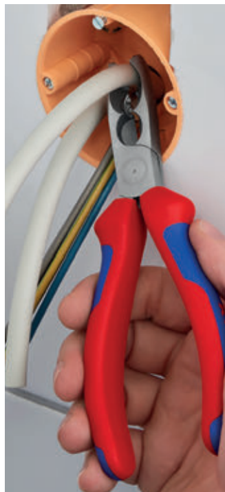
Abmanteln tief unten in der Unterputzdose
