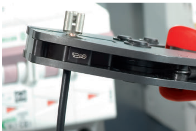
Gut sichtbare Kennzeichnung der Crimpeinsätze mit Piktogrammen
