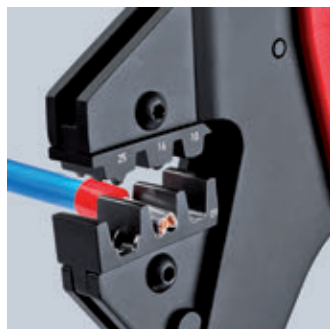
97 43 200 mit Crimpeinsatz 97 49 09 für Aderendhülsen
